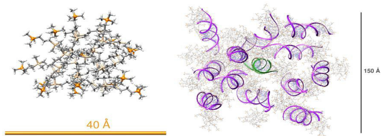
Obrázek 1: Počítačový model kationického karbosilanového dendrimery (3. generace) s fosfoniovými (PMe3) koncovkami (vlevo) a nasimulovaný dendriplex sestávající ze 36 těchto endrimerů a 13 siRNA molekul (vpravo). V obou případech se jedná o výsledky simulací ve vodném prostředí.
