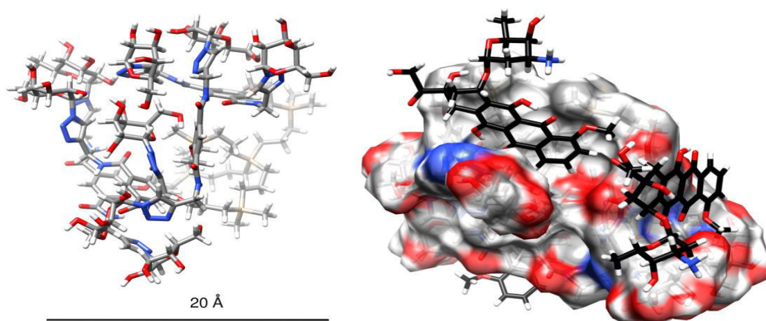
Obrázek 2: Počítačový model karbosilanového dendrimery (1. generace) s galktózovými koncovkami (vlevo) a nasimulovaný komplex tohoto dendrimery a 3molekul doxorubicinu (vpravo). V obou případech se jedná o výsledky simulací ve vodném prostředí.
